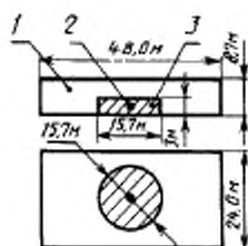
1 - помещение; 2 - аппарат; 3 - взрывоопасная зона
